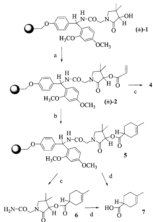
Scheme 1. Reagents: (a) acryloyl chloride, \text{NEt}_3 , \text{CH}_2\text{Cl}_2 ; (b) \text{CH}_2\text{Cl}_2 , \text{TiCl}_4 , isoprene; (c) TFA, \text{CH}_2\text{Cl}_2 ; (d) \text{LiOH} , \text{H}_2\text{O} , THF
